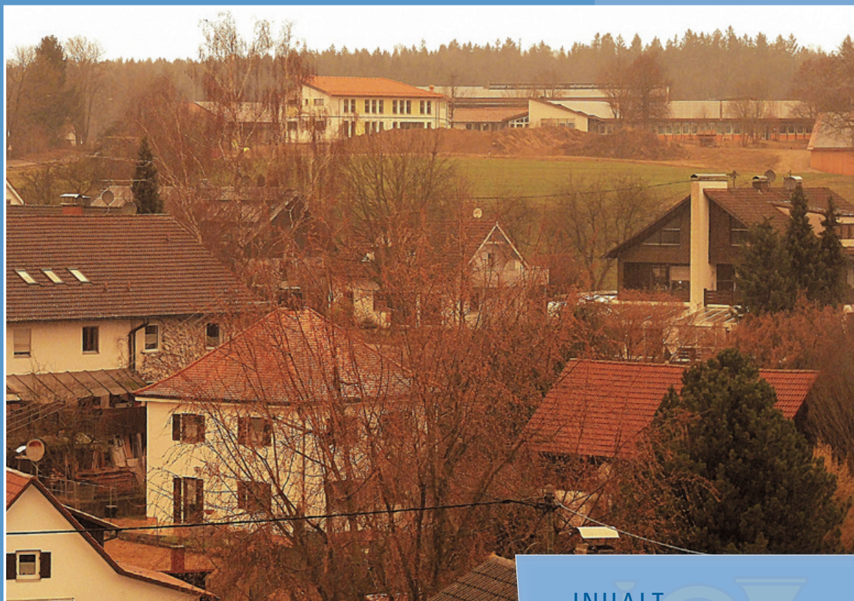
Saharastaub am 15. März 2022
